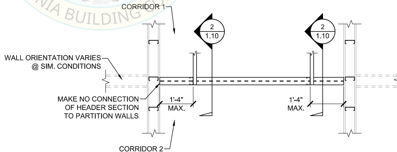
1 ENLARGED SYSTEM SEPARATION PLAN SCALE: N.T.S.
