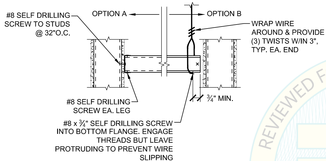
3 SPREADER/TRAPEZE END CONNECTIONS SCALE: N.T.S.
