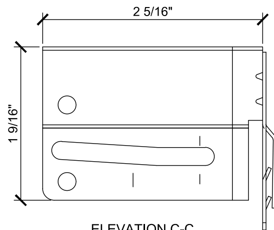
ELEVATION C-C
