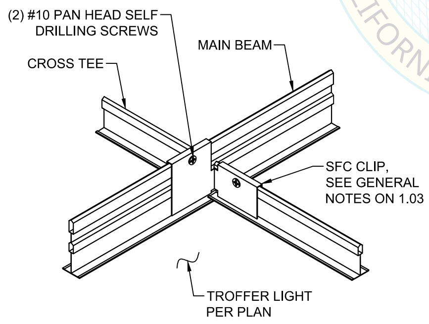
3 CONNECTION @ TROFFER LIGHTS SCALE: N.T.S.
