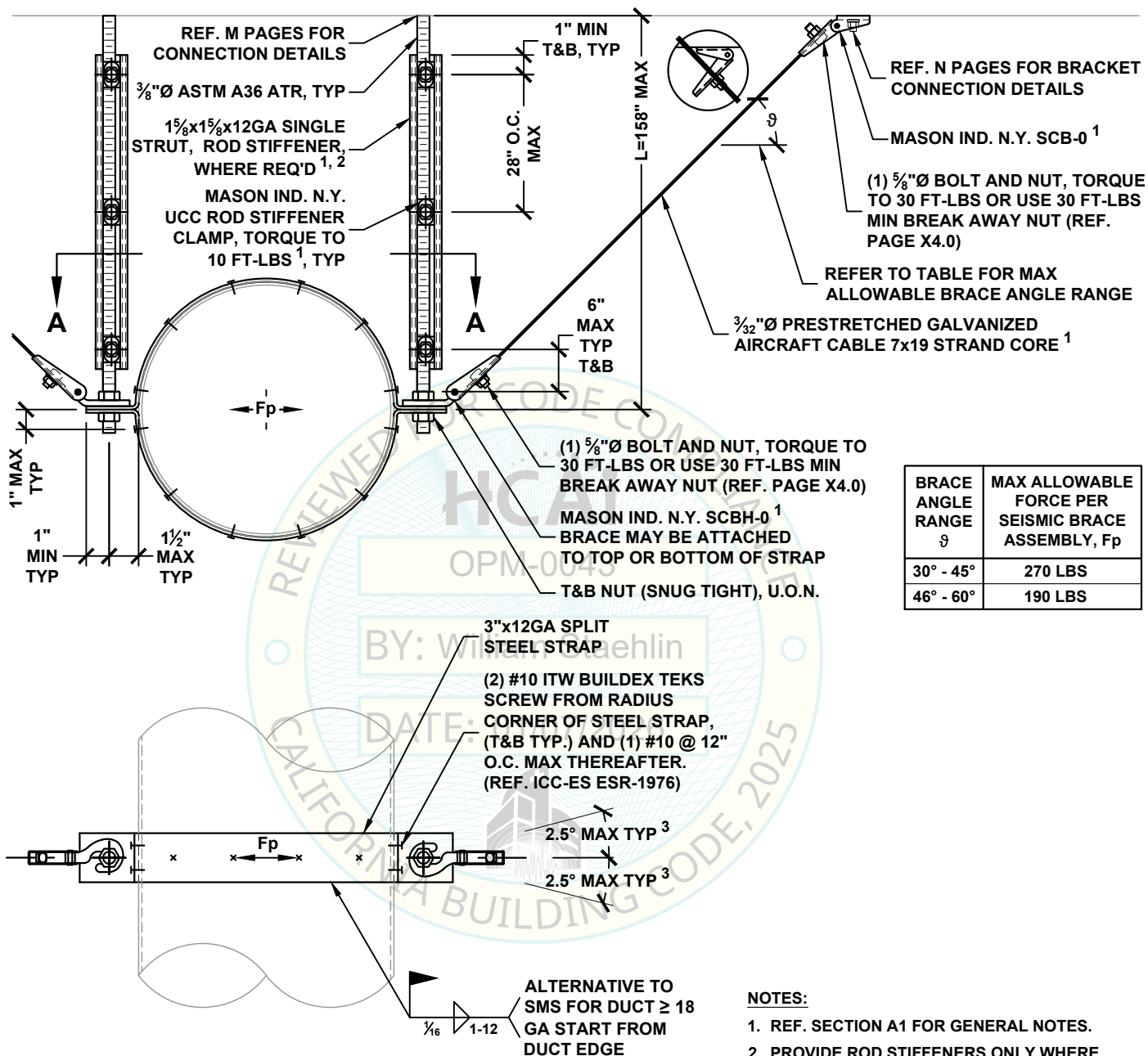
VIEW A-A
