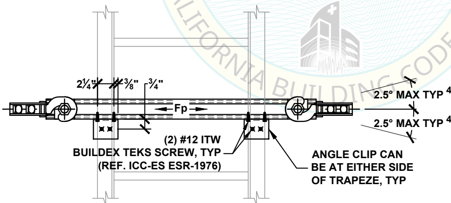
VIEW A-A
