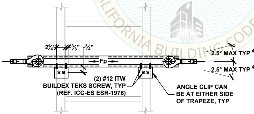
VIEW A-A
