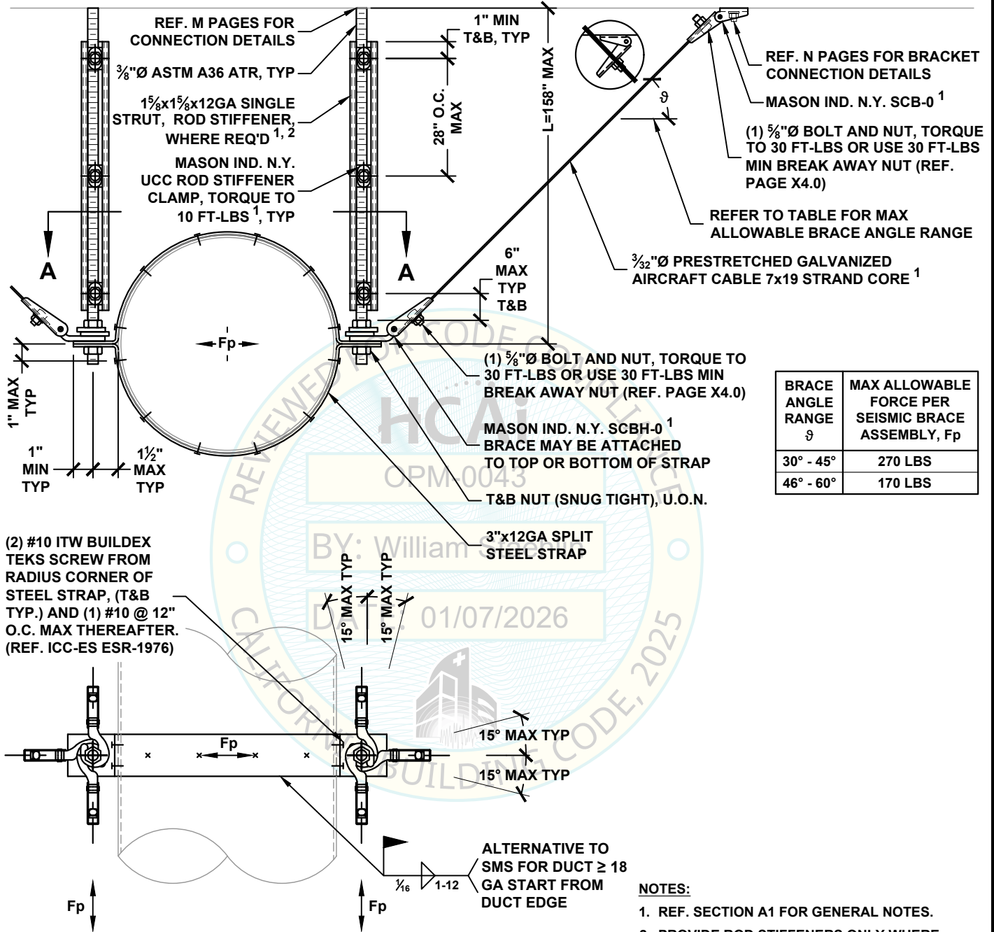
VIEW A-A
