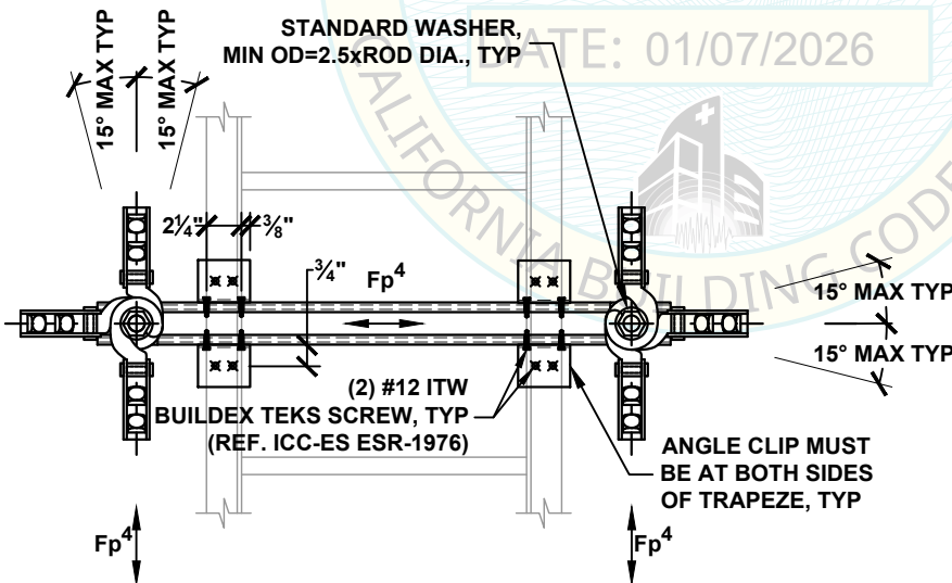
VIEW A-A
