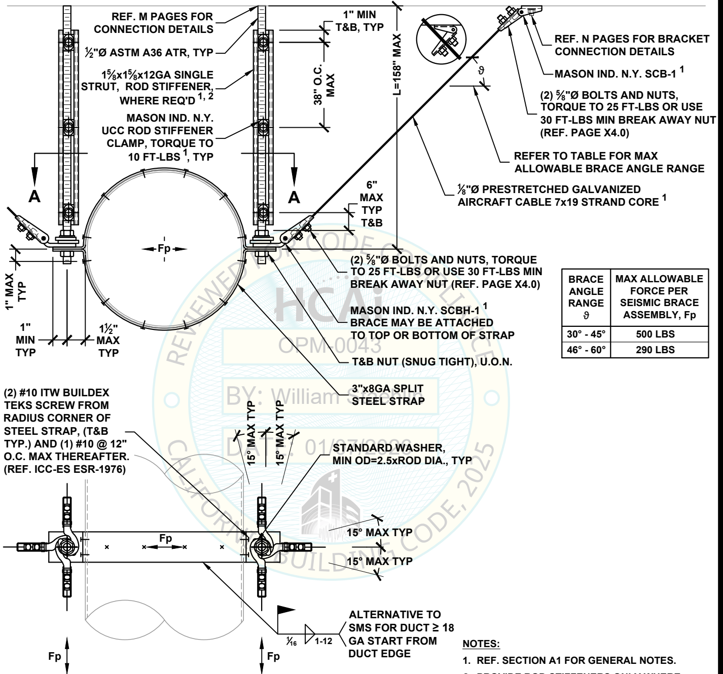
VIEW A-A
