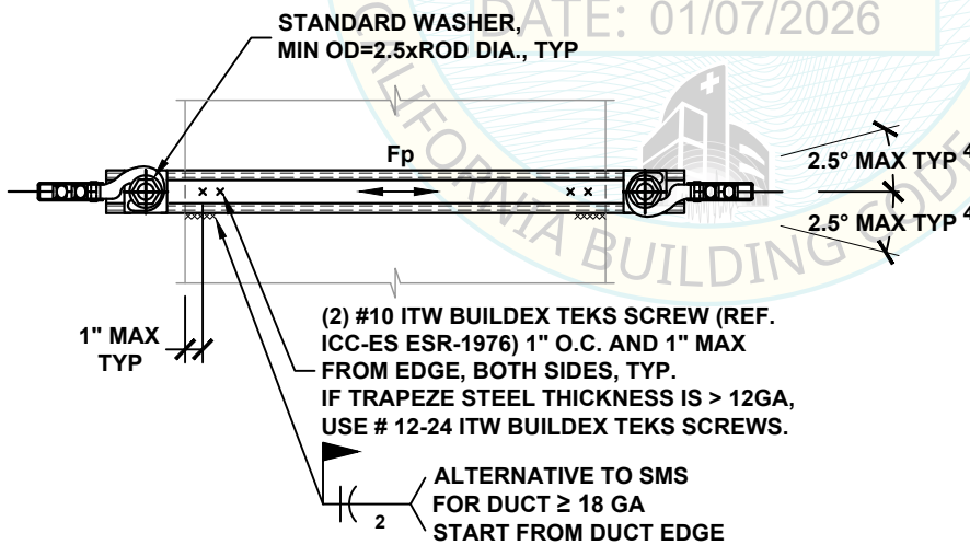
VIEW A-A
