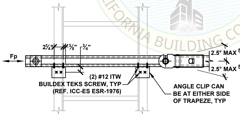
VIEW A-A
